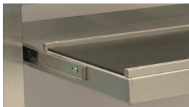
スライド棚(導電ゴムシート貼り)
